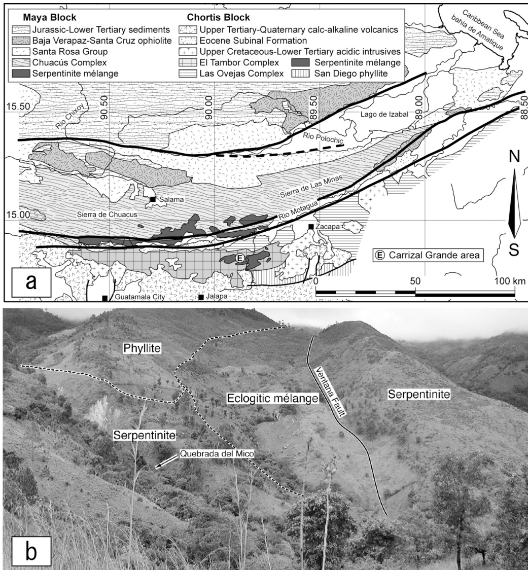
図 1. (a) グアテマラ中央部モタグア断層帯の地質図. Tsujimori et al. (2006a) を改図. (b) モタグア断層帯南部カリザルグランデ地域のローソン石エクロジイトを含む蛇紋岩メランジュの風景.
