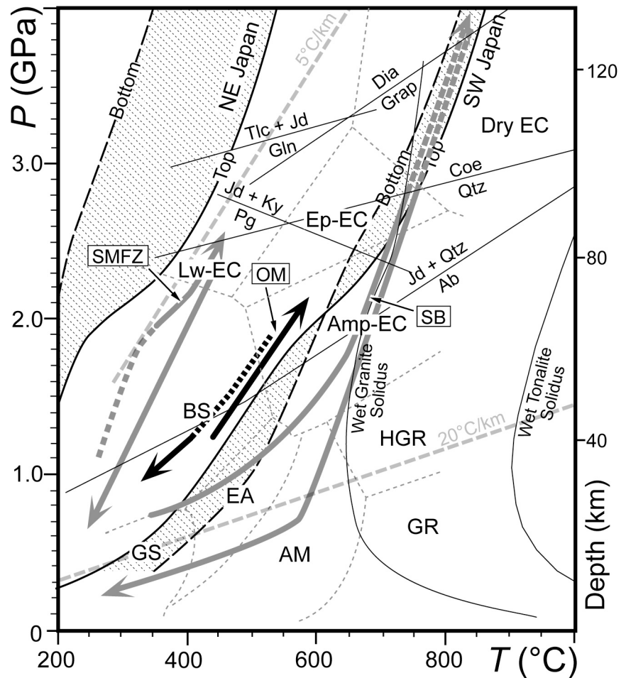
図3. 青海(OM)の藍閃石-緑れん石エクロジヤイトの変成経路を示した圧力(P)-温度(T)図(辻森・松本, 2006)。比較のためモタグア断層帯のローソン石エクロジヤイト(SMFZ: Tsujimori et al. , 2006a), 及び三波川帯のエクロジヤイト(SB: Ota et al. , 2004)の変成経路を示した。変成相の略号とその境界線, 及び主要な反応曲線の位置はLiou et al. (2004)による。斜線の領域は現在の東北日本と西南日本に沈み込むスラブ上面・下面に予測される温度構造(Peacock and Wang, 1999)を表す。
