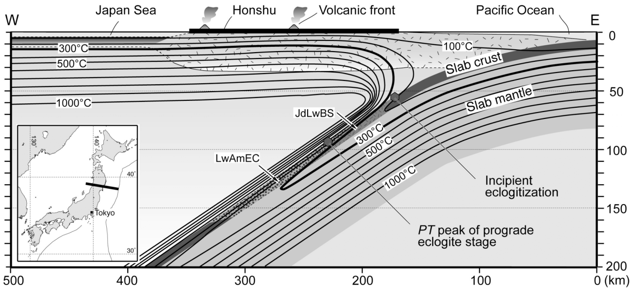
図 4. 現在の東北日本直下に予測される温度構造とモタグア断層帯のローソン石エクロジヤイトから推定されるエクロジヤイト化と変成ピークの圧力・温度の位置関係. Hacker et al. (2003a) の前進モデリングによる岩石学的構造も示した.
